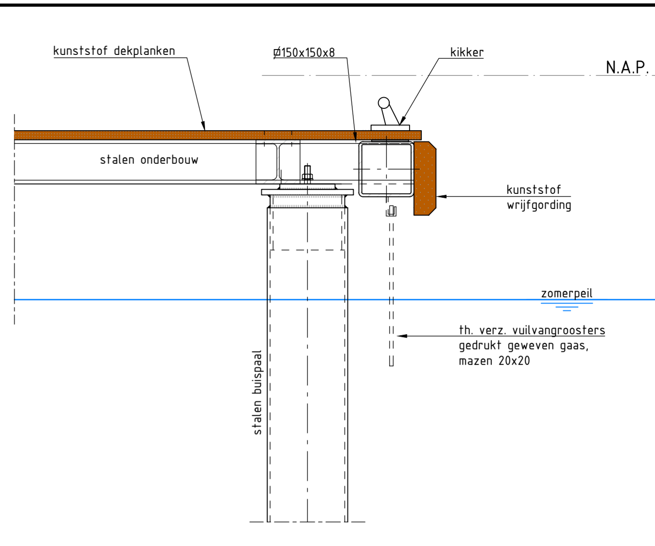
PRINCIPE DETAIL 1: STEIGER ELEMENT OP PALEN SCHAAL 1:10
