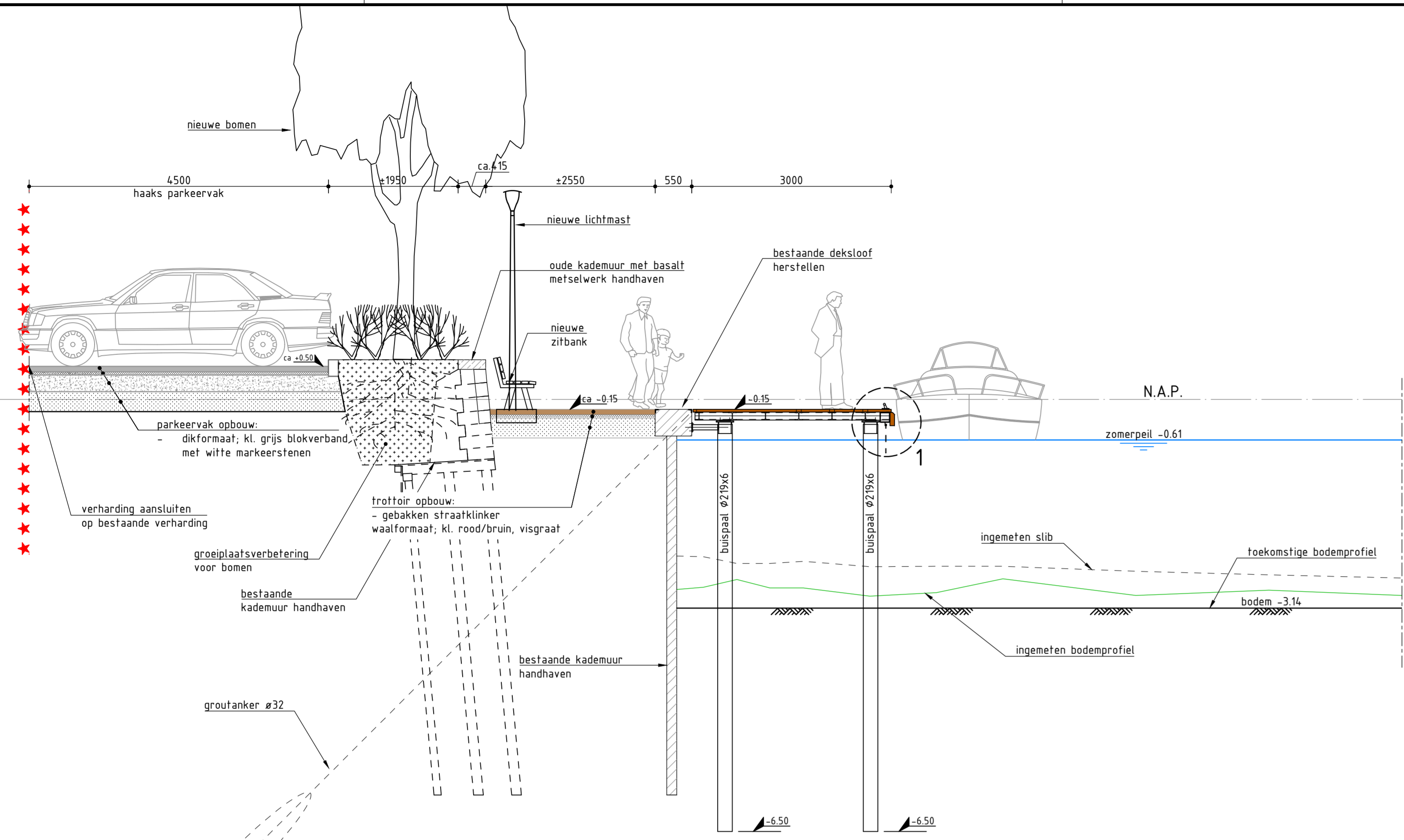
DOORSNEDE A-A SCHAAL 1:50 Inrichting Havenstraat en steiger Havenstraat
